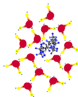
Agregación de lípidos en medio acuoso
