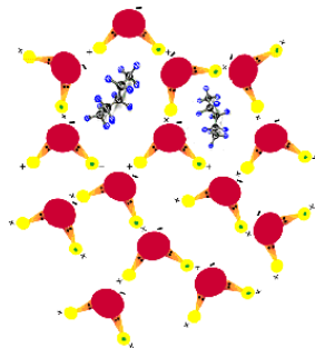
Dispersión de lípidos en medio acuoso
